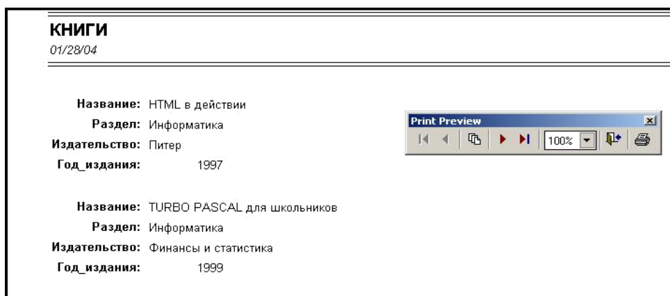
Рисунок 13.8. Отчёт Книги
