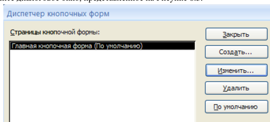
Рисунок 8.3. Диспетчер кнопок
