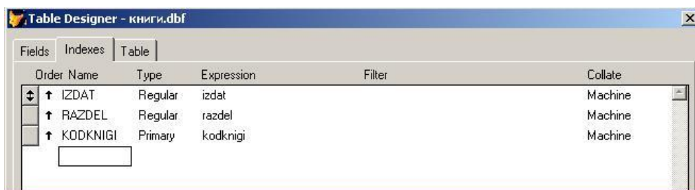
Рисунок 9.5. Вкладка Indexes (Индексы) окна TableDesigner таблицы Книги Индекс, с присвоенным типом Primary является первичным ключом таблицы 9. Аналогично внести изменения в таблицы БД Библиотека: Разделы, Издательство, Автор_книги, Авторы в соответствии с таблицами 9.16,9.17, 9.18, 9.19 Таблица 9.16.Определение индексов таблицы Разделы на вкладке Indexes (Индексы) окна конструктора таблицы TableDesigner
