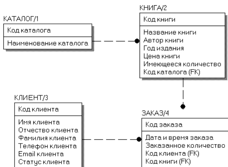
Рисунок 14.1. Логическая модель данных предметной области
