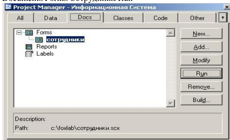
Рисунок 10.6. Окно ProjectManager
