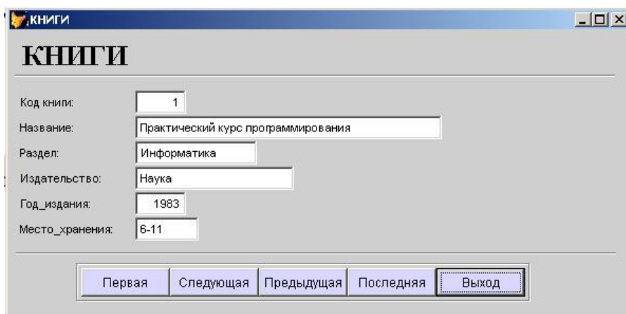
Рисунок 10.12. Форма Книги
