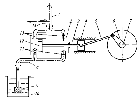
Рисунок 1 - Схема работы двухцилиндрового бурового насоса:
